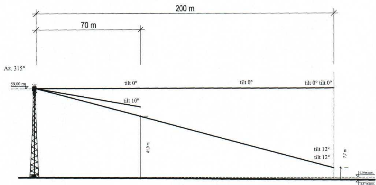
Rys. 4. Rzut pionowy osi głównej wiązki promieniowania na azymucie 315° w odległości 70 i 200 metrów od środka elektrycznego anteny sektorowej dla tiltów 0°, 10° oraz 12°.
