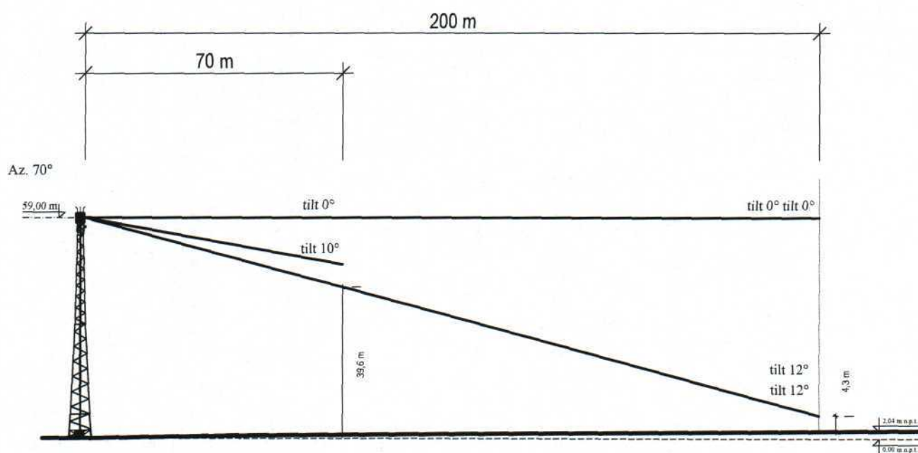
Rys. 2. Rzut pionowy osi głównej wiązki promieniowania na azymucie 70° w odległości do 70 i 200 metrów od środka elektrycznego anteny sektorowej dla tiltów 0°, 10° oraz 12°.
