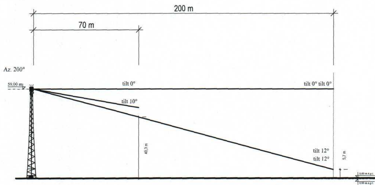
Rys. 3. Rzut pionowy osi głównej wiązki promieniowania na azymucie 200° w odległości 70 i 200 metrów od środka elektrycznego anteny sektorowej dla tiltów 0°, 10° oraz 12°.
