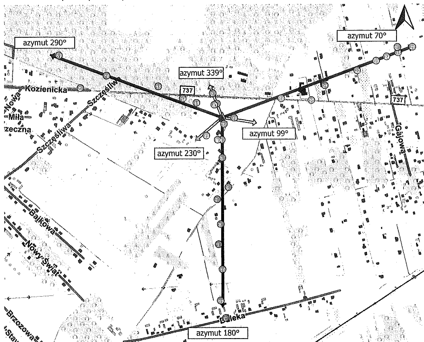
Załącznik 2. Widok pionów pomiarowych
